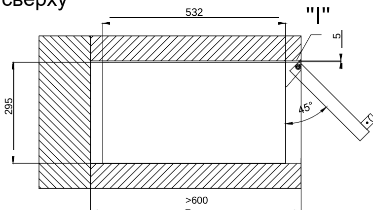
Вид сверху
