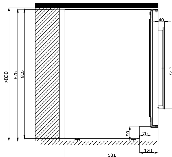
Вид сбоку
