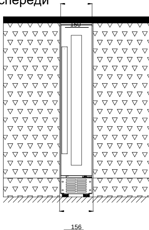
Вид спереди
