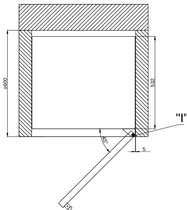
Вид сверху
