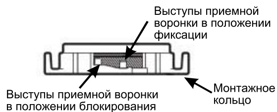
Фиксация детали
